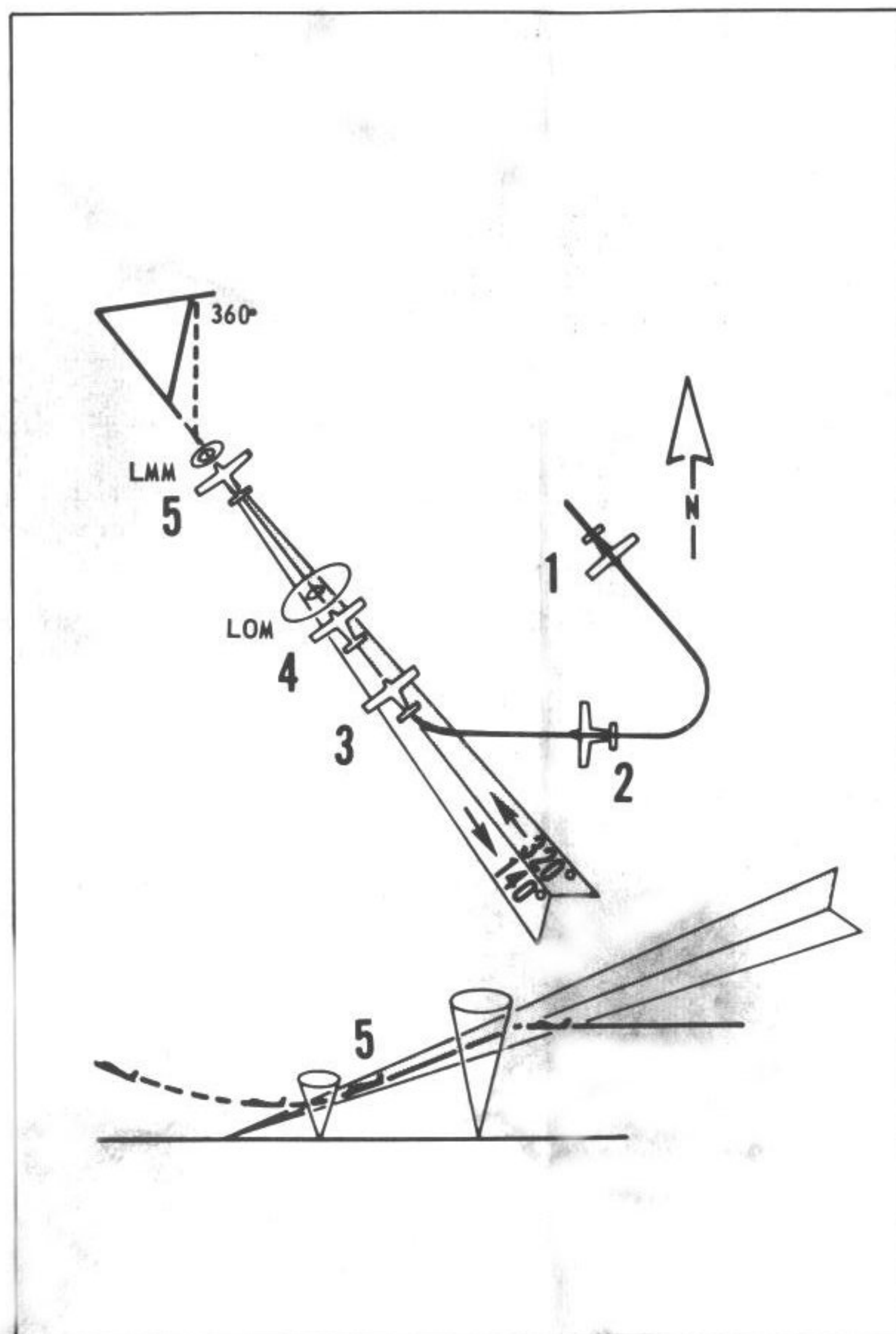
ILS FRONT COURSE APPROACH
