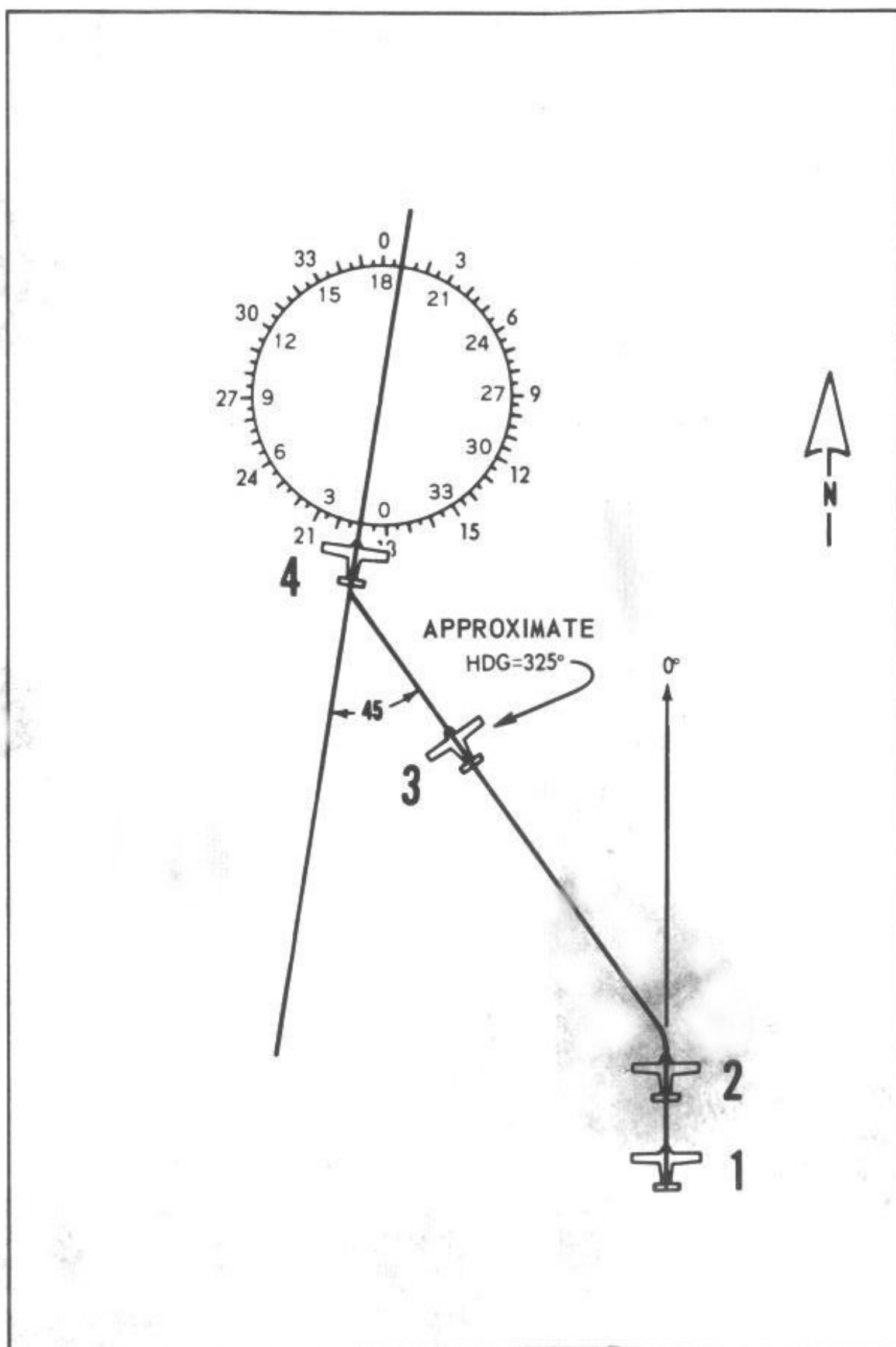
INTERCEPTING VOR RADIAL
